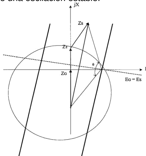
FIGURA 9.20 Detector mho de pérdida de sincronismo con blinders.
