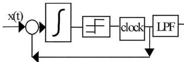
FIGURA 9.38 Modulador Signa-Delta.
