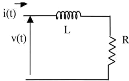
FIGURA 9.40 Modelo de una línea con falla.
