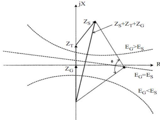
FIGURA 9.19 Locus de impedancia para diferentes ángulos de fuente.
