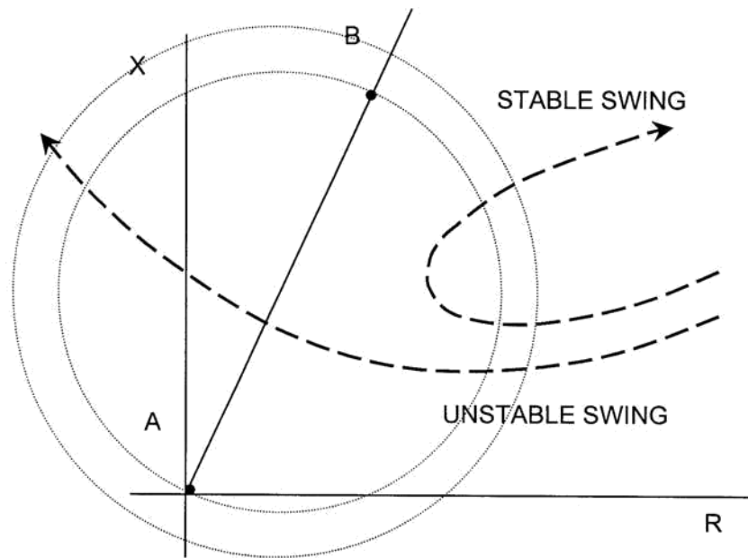
FIGURA 9.34 Trayectorias de oscilaciones estables e inestables en el plano de impedancia.
