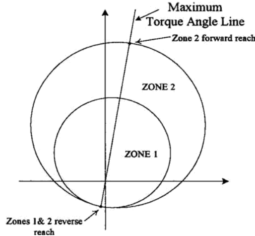
FIGURA 9.17 Aplicación típica de elementos 21.
