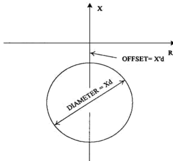
FIGURA 9.8 Pérdida de excitación offset-mho característica.
