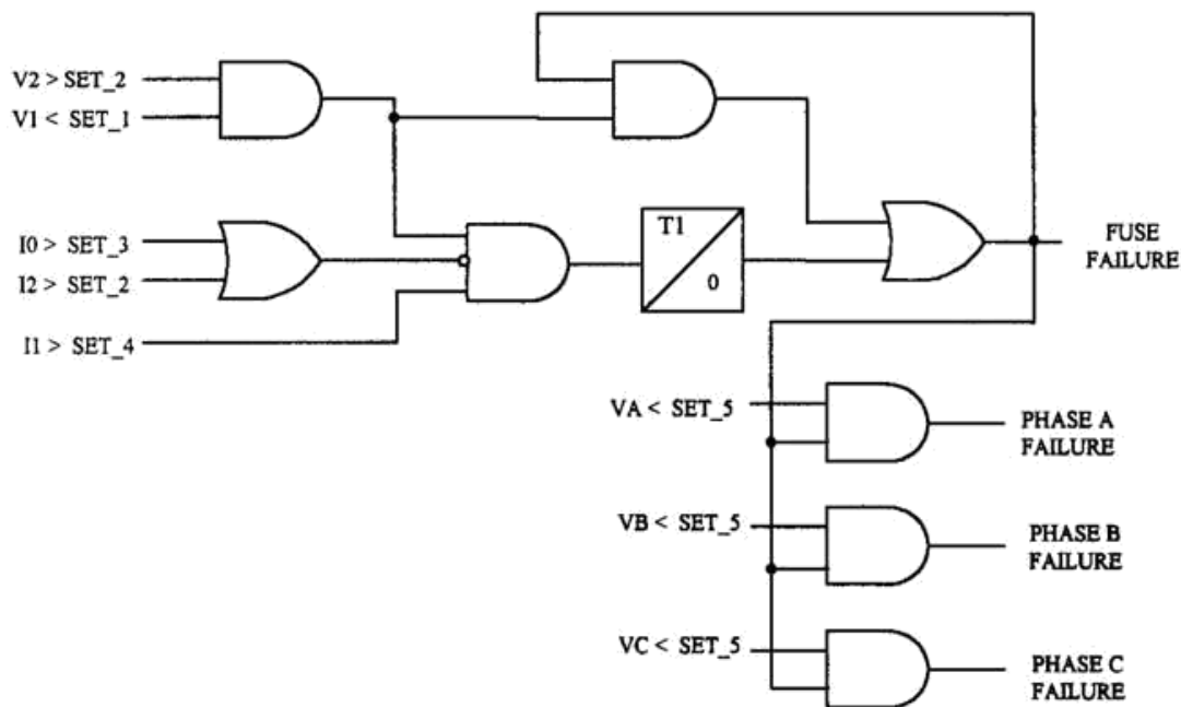
FIGURA 9.14 Implementación de las componentes simétricas en la detección de falla de fusible.
