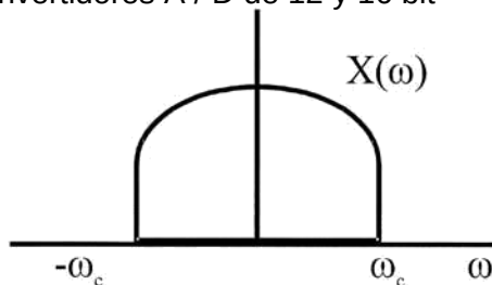
FIGURA 9.35 La Transformada de Fourier de una función de banda limitada.
