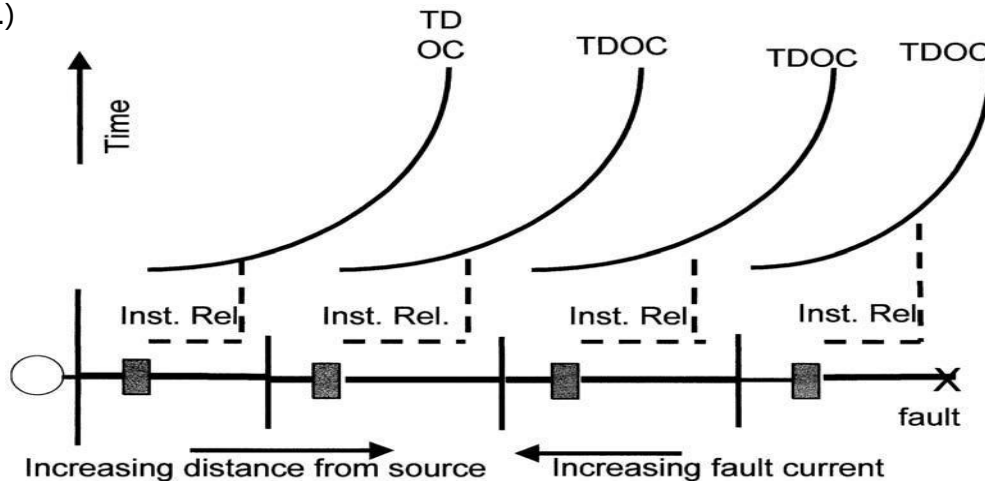
FIGURA 9.31 Efecto de relés instantáneos. ( Fuente: Horowitz, SH y Phadke, AG, Retransmisión del sistema de potencia , 2ª ed., 1995. Research Studies Press, Reino Unido Con permiso.)
