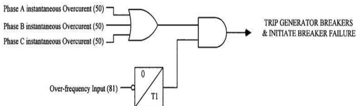
FIGURA 9.23 Protección contra energización inadvertida por sobrecorriente supervisada por frecuencia.
