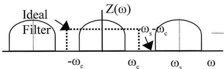
FIGURA 9.36 La Transformada de Fourier de una versión muestreada de la señal x(t) .
