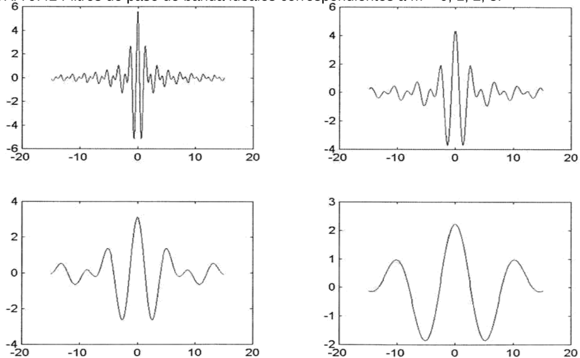
FIGURA 9.43 Las respuestas de impulso correspondientes a los filtros en Fig. 9.42.
