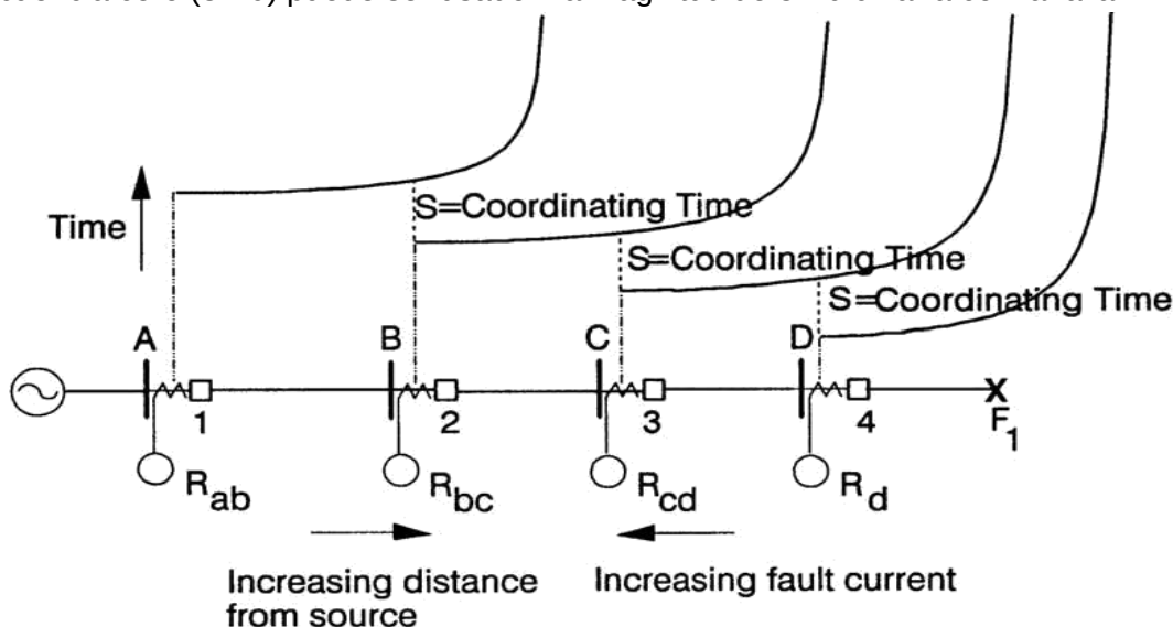
FIGURA 9.30 Coordinación de relés TDOC. ( Fuente: Horowitz, SH y Phadke, AG, Retransmisión del sistema de potencia , 2ª ed., 1995. Research Studies Press, Reino Unido Con permiso.)
