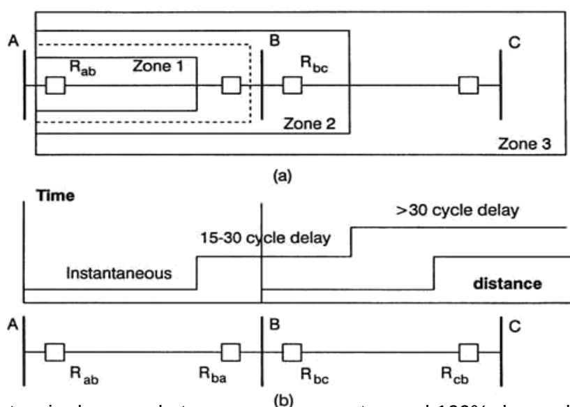
FIGURA 9.33 Distancia de paso de tres zonas para proteger el 100% de una línea y respaldar la línea vecina. (Fuente: Horowitz, SH y Phadke, AG, Retransmisión del sistema de potencia , 2ª ed., 1995. Research Studies Press, Reino Unido Con permiso.)
