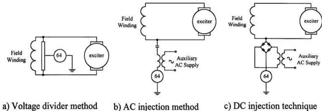
FIGURA 9.7 Diversas técnicas para la protección del terreno.
