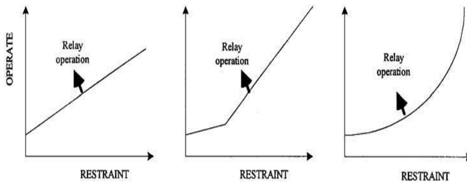
FIGURA 9.3 Características diferenciales de porcentaje de pendiente simple, doble y variable.
