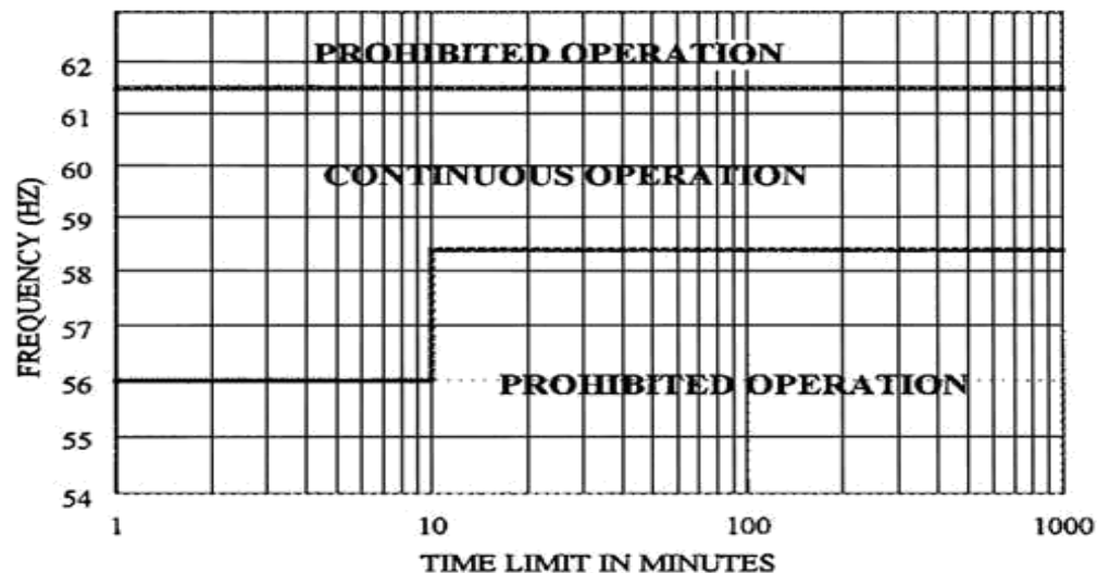
FIGURA 9.22 Característica típica de protección de frecuencia anormal.
