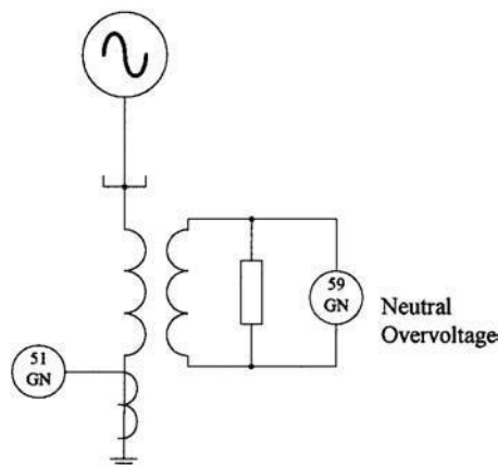
FIGURA 9.5 Esquema de sobretensión neutral de estator a tierra.
