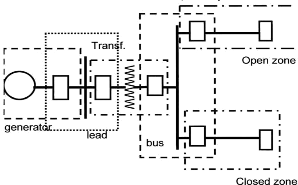
FIGURA 9.26 Zonas de protección cerradas y abiertas. ( Fuente: Horowitz, SH y Phadke, AG, Retransmisión del sistema de potencia , 2ª ed., 1995. Research Studies Press, Reino Unido Con permiso.)
