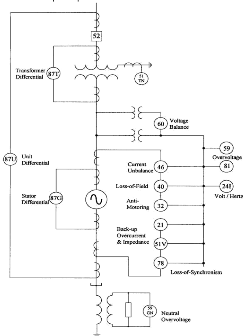
FIGURA 9.2 Esquema típico de protección generador-transformador.
