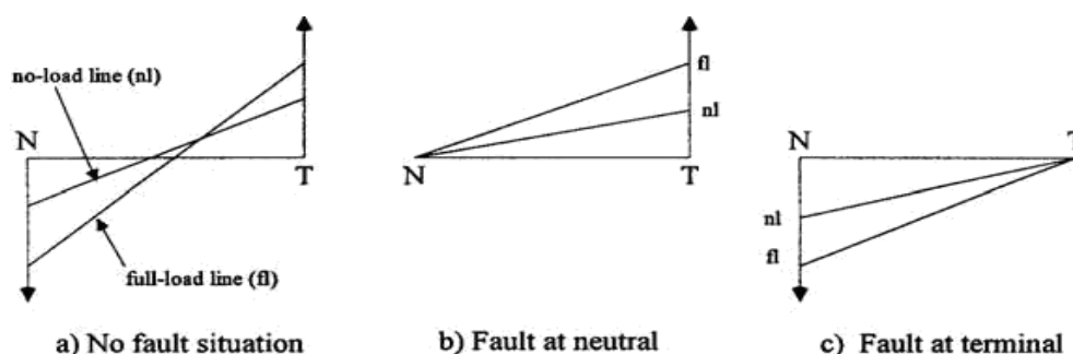
FIGURA 9.6 Tercer armónico en el neutro y terminales.
