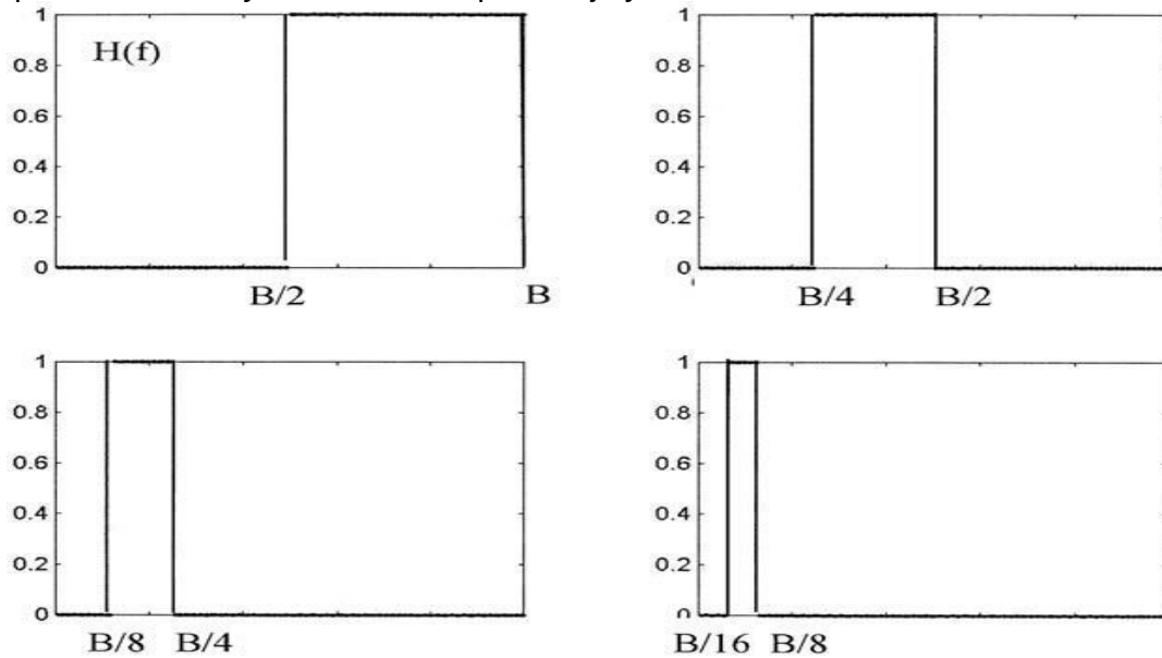
FIGURA 9.42 Filtros de paso de banda ideales correspondientes a m = 0, 1, 2, 3 .
