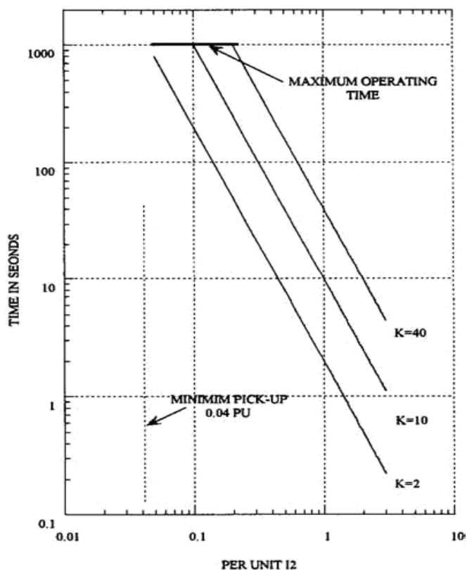
FIGURA 9.10 Típica curva estática o digital de tiempo inverso 46.
