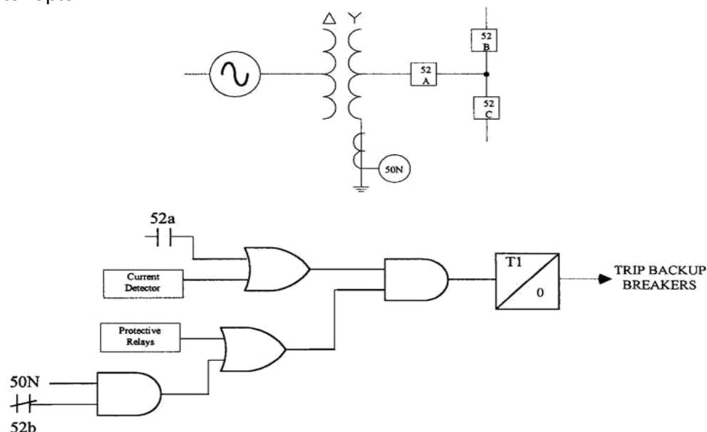
FIGURA 9.24 Lógica de falla del interruptor con protección antideslumbrante.
