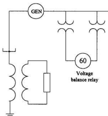
FIGURA 9.13 Ejemplo de relé de equilibrio de tensión.
