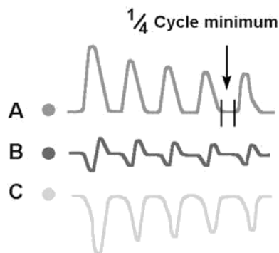
FIGURA 9.1 Formas de onda de corriente de entrada del transformador.
