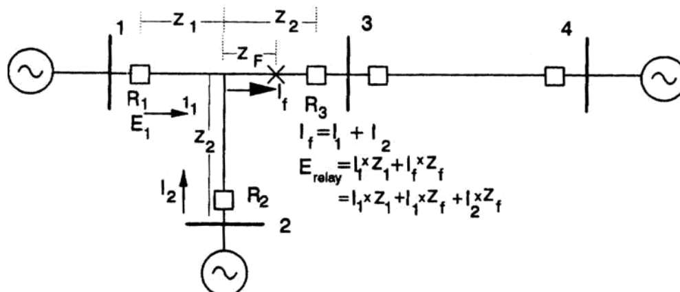
FIGURA 9.27 Efecto de la alimentación en los relés locales. ( Fuente: Horowitz, SH y Phadke, AG, Retransmisión del sistema de potencia , 2ª ed., 1995. Research Studies Press, Reino Unido Con permiso.)
