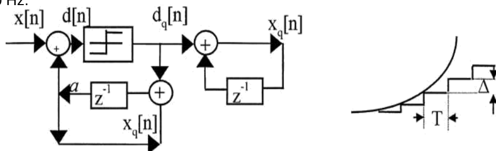
FIGURA 9.37 Modulador Delta y error.
