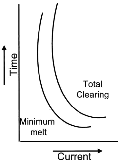
FIGURA 9.28 Fusible tiempo-corriente característica. (Fuente: Horowitz, SH y Phadke, AG, Retransmisión del sistema de potencia , 2ª ed., 1995. Research Studies Press, Reino Unido Con permiso.)
