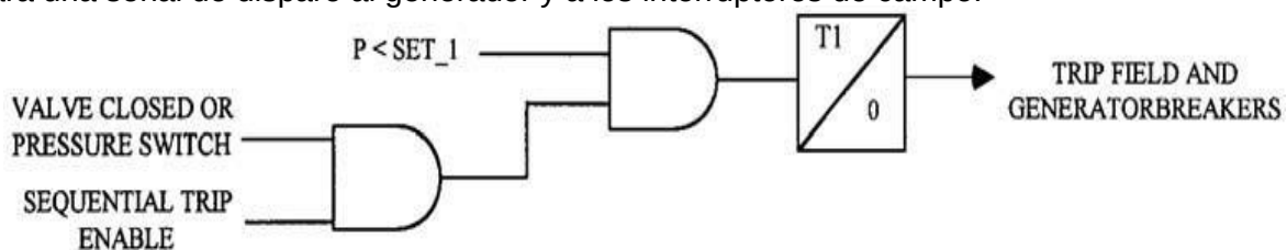
FIGURA 9.25 Implementación de una función de disparo secuencial.
